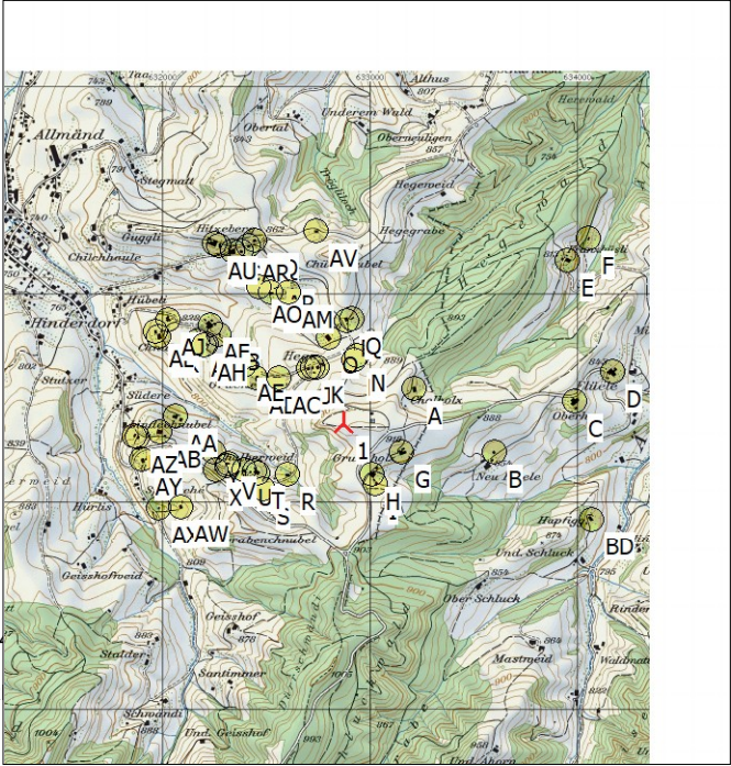
Maßstab 1:40 ' 000 Neue WEA Schattenrezeptor
